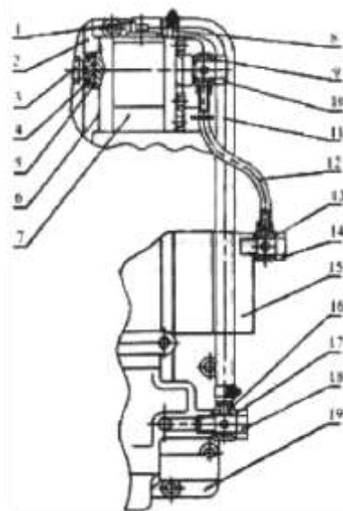
Рис. 3.33. Гидравлическая система.
