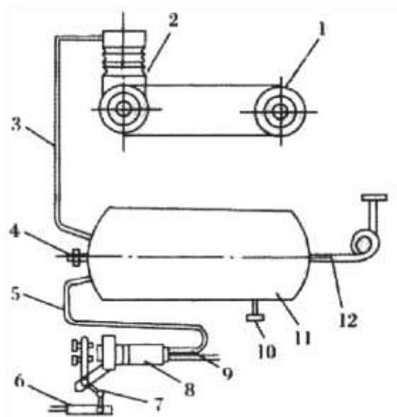
Рис. 3.18. Структура пневмотормоза.
