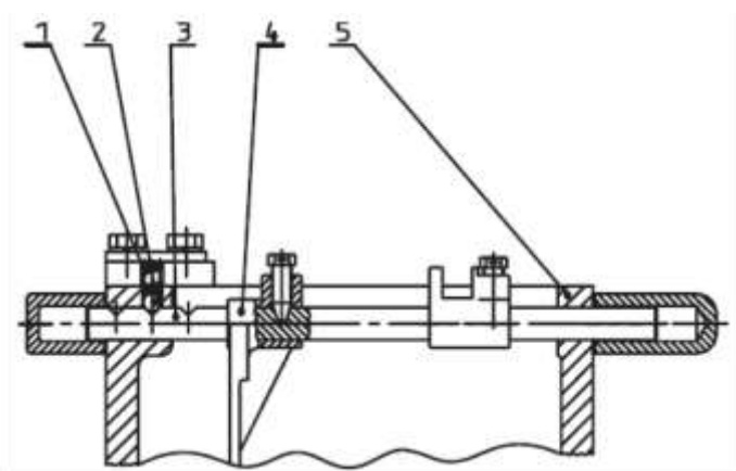
Рис. 3.11. Блокировочный механизм.
